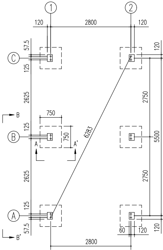
基礎伏図 (S= 1/80)
