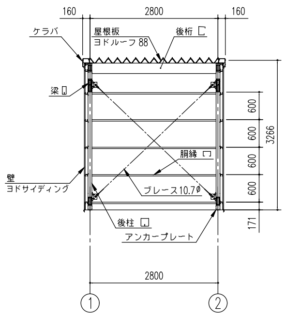
正面断面図 (S= 1/80)
