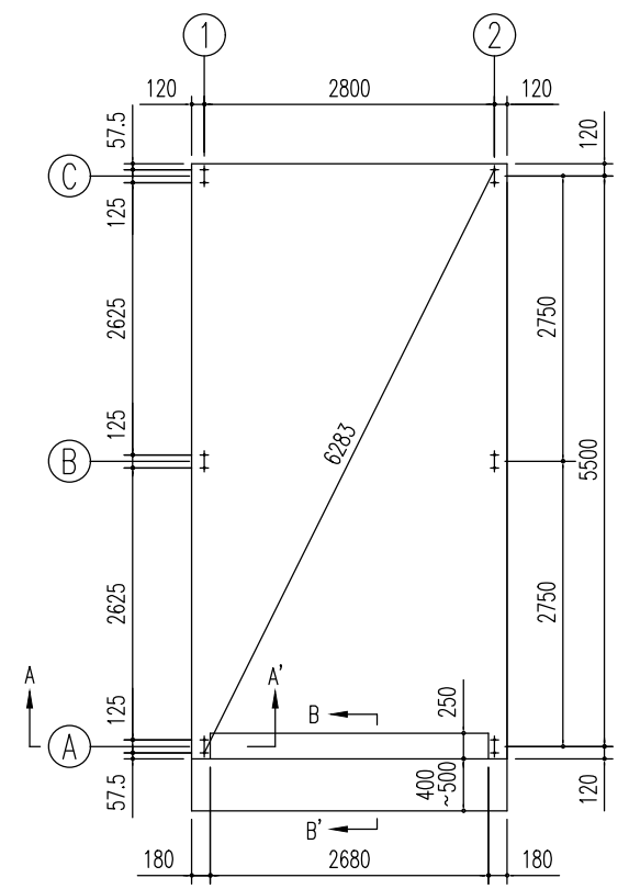
基礎伏図 (S= 1/80)
