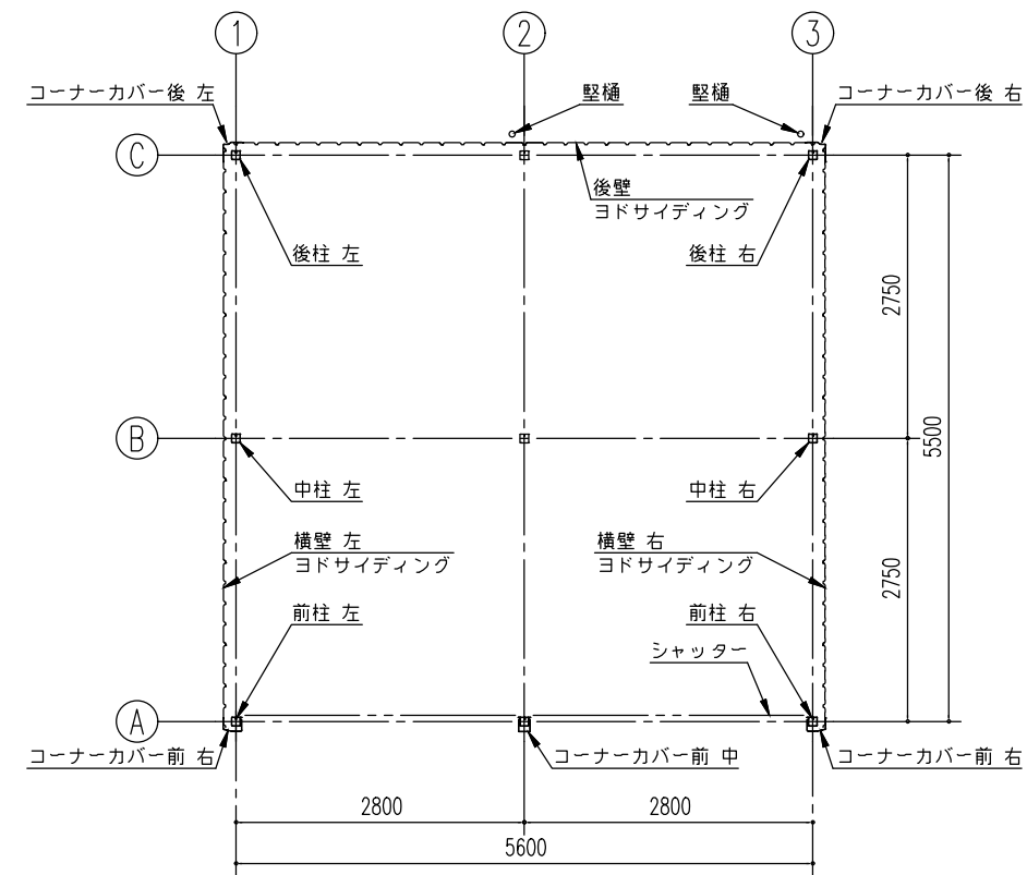
平面図 (S=1/80)
