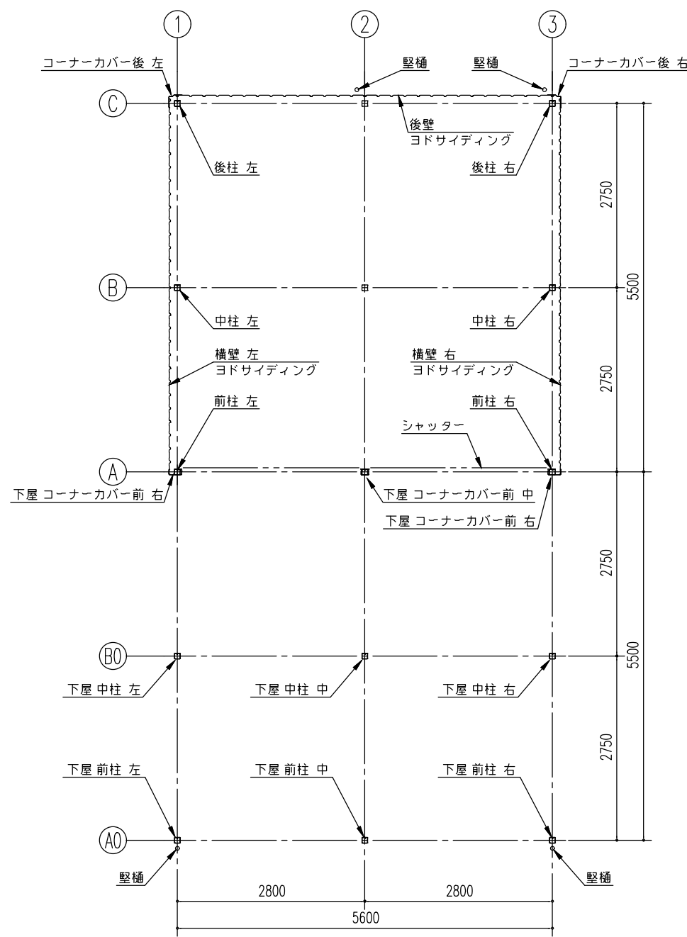
平面図 (S=1/80)
