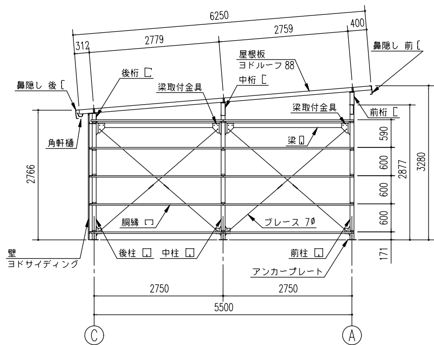
側面断面図 (S= 1/80) ※側面の出入口により、ブレースの配置が変更となる場合があります。
