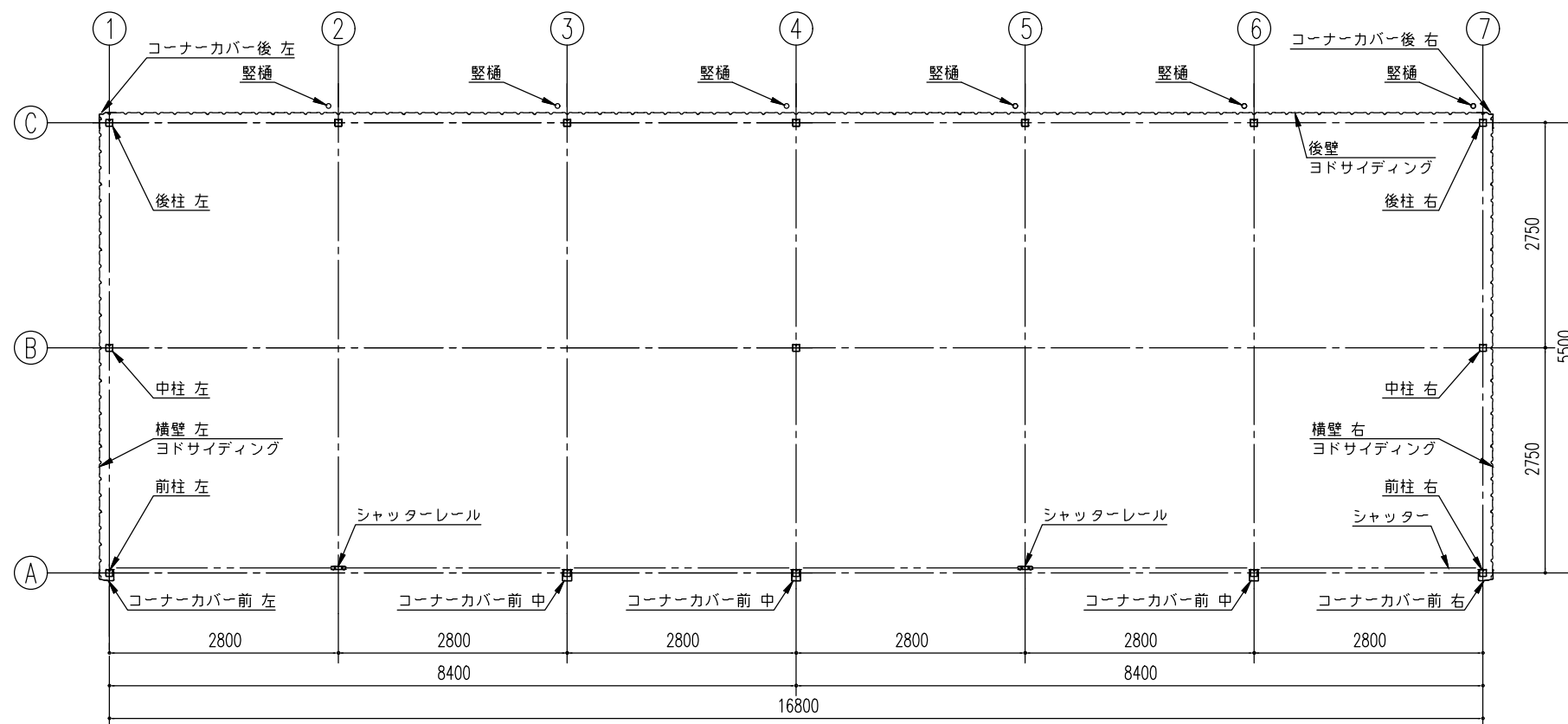
平面図 (S=1/80)
