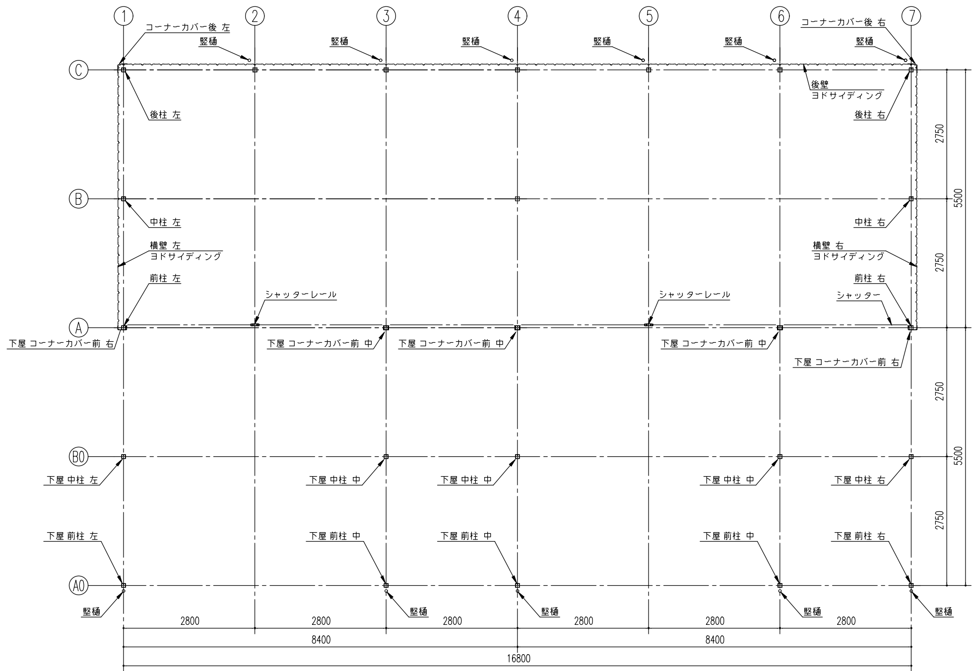
平面図 (S= 1/80)
