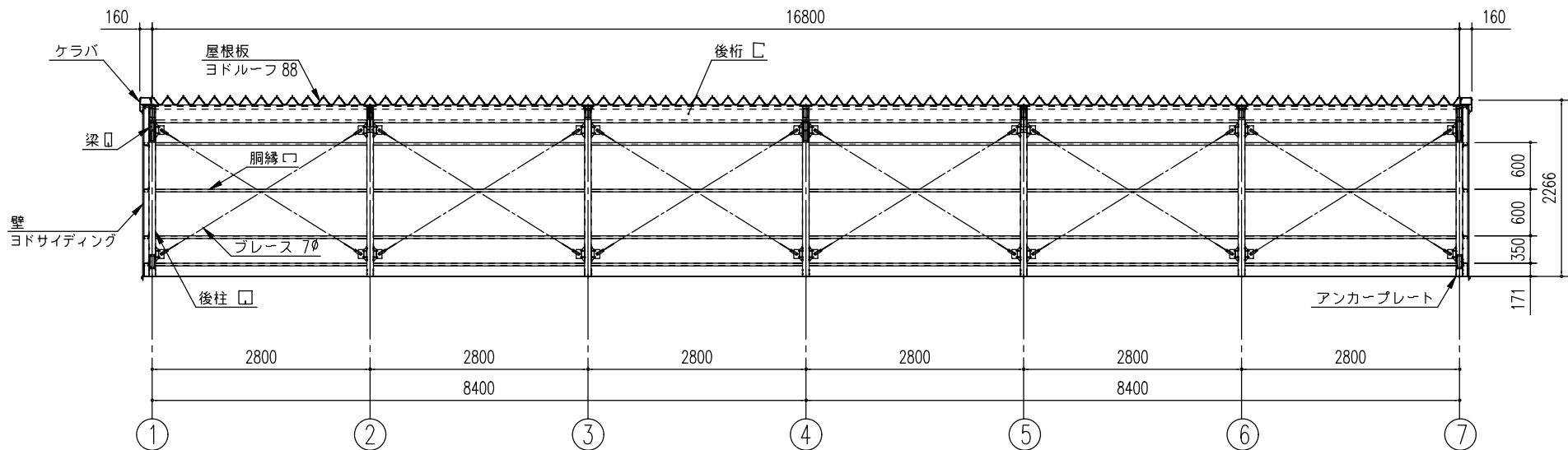
正面断面図 (S= 1/80)
