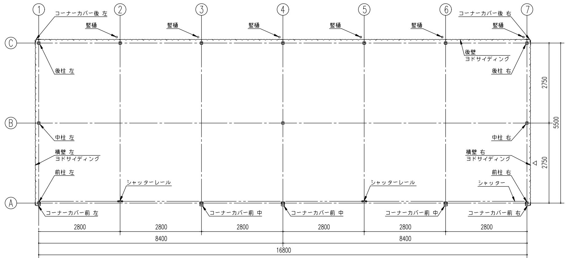
平面図 (S=1/80)
