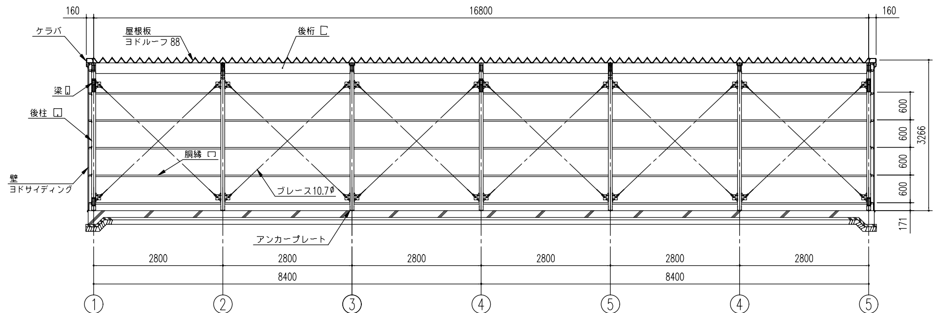
本体 正面断面図 (S=1/80)
