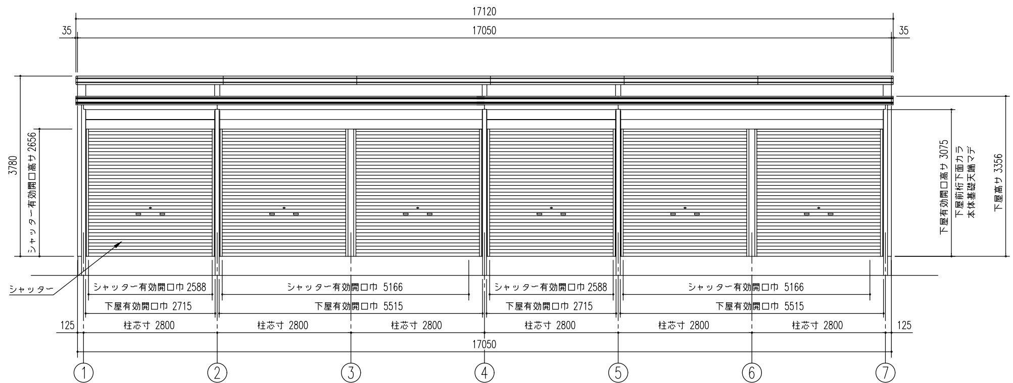
正面立面図(S= 1/80)
