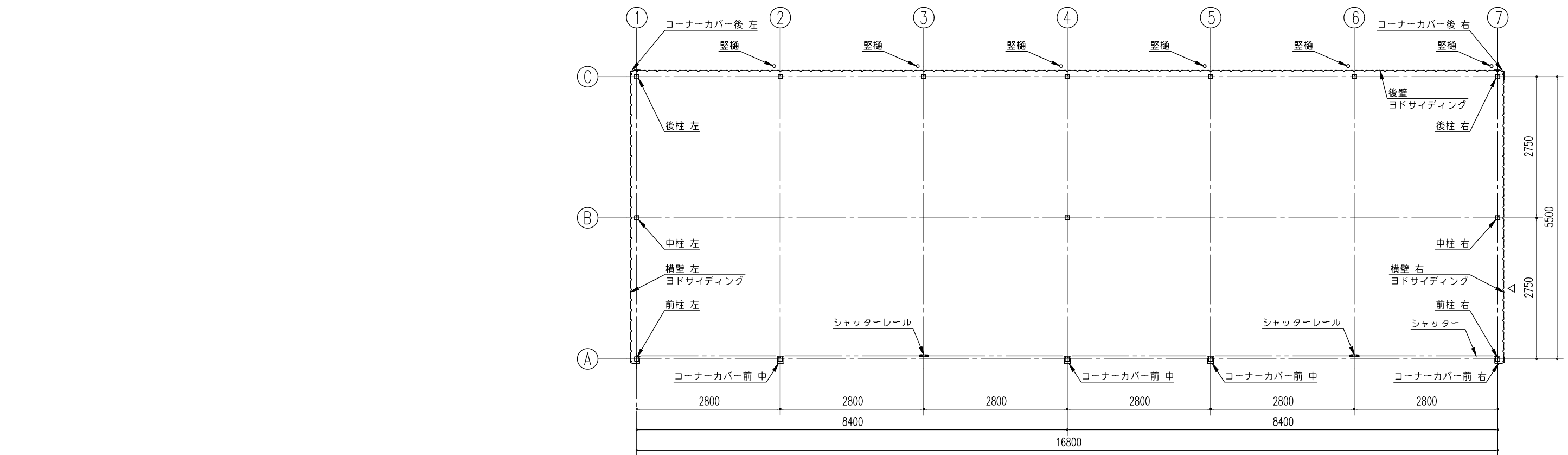
平面図 (S= 1/80)
