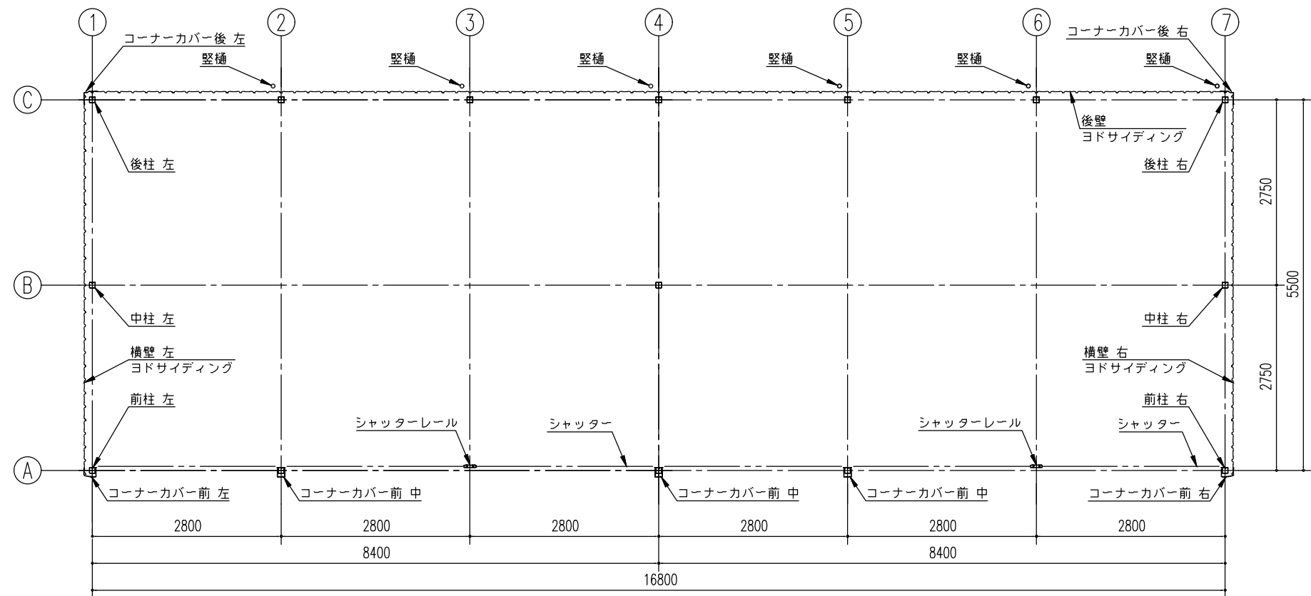
平面図(S=1/80)
