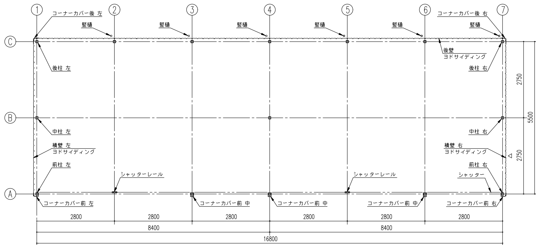
平面図 (S= 1/80)
