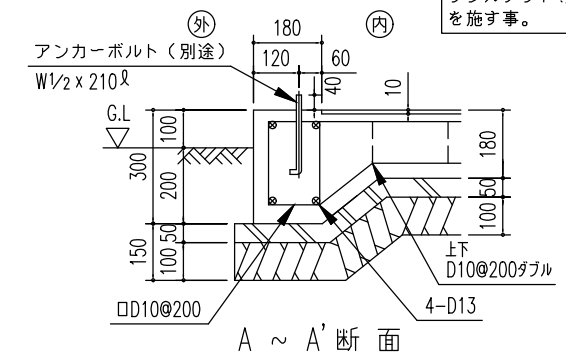
埋金具詳細図 (S=1/20)
