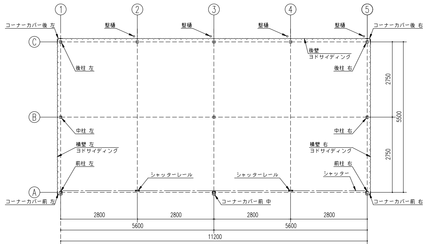
平面図 (S=1/80)
