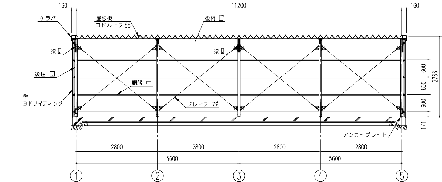
本体 正面断面図 (S= 1/80)
