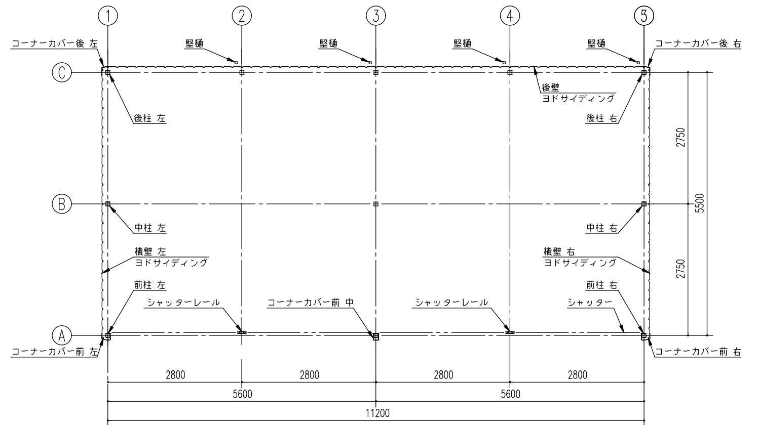
平面図 (S= 1/80)
