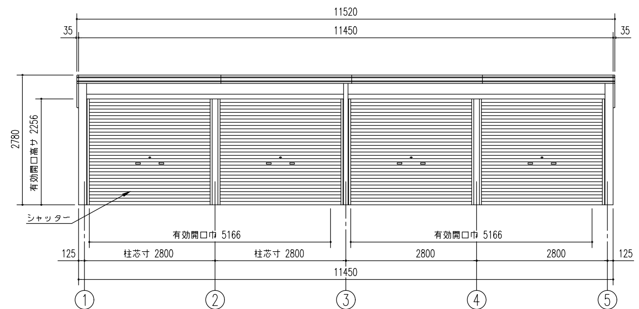
正面立面図(S= 1/80)
