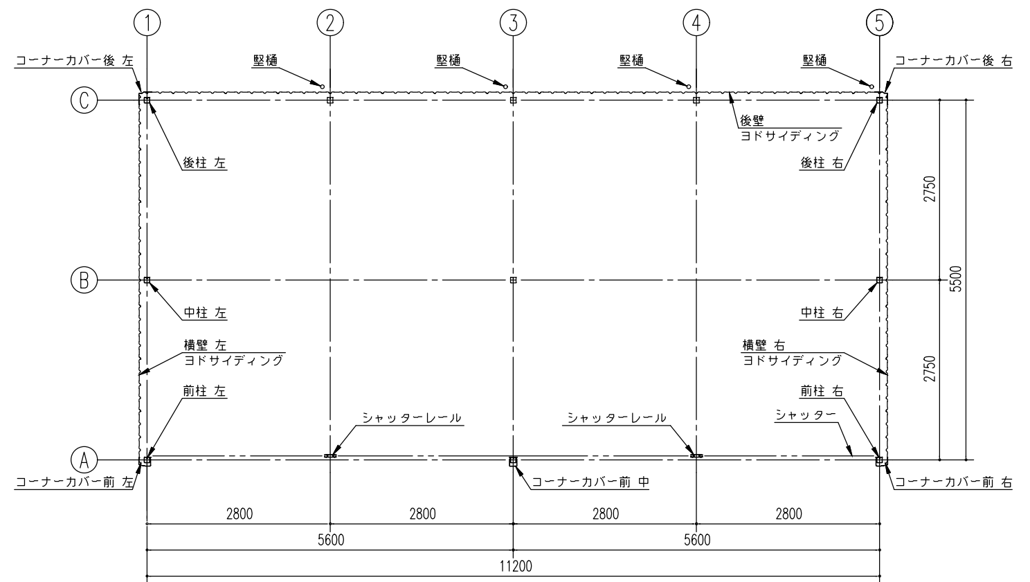
平面図 (S=1/80)
