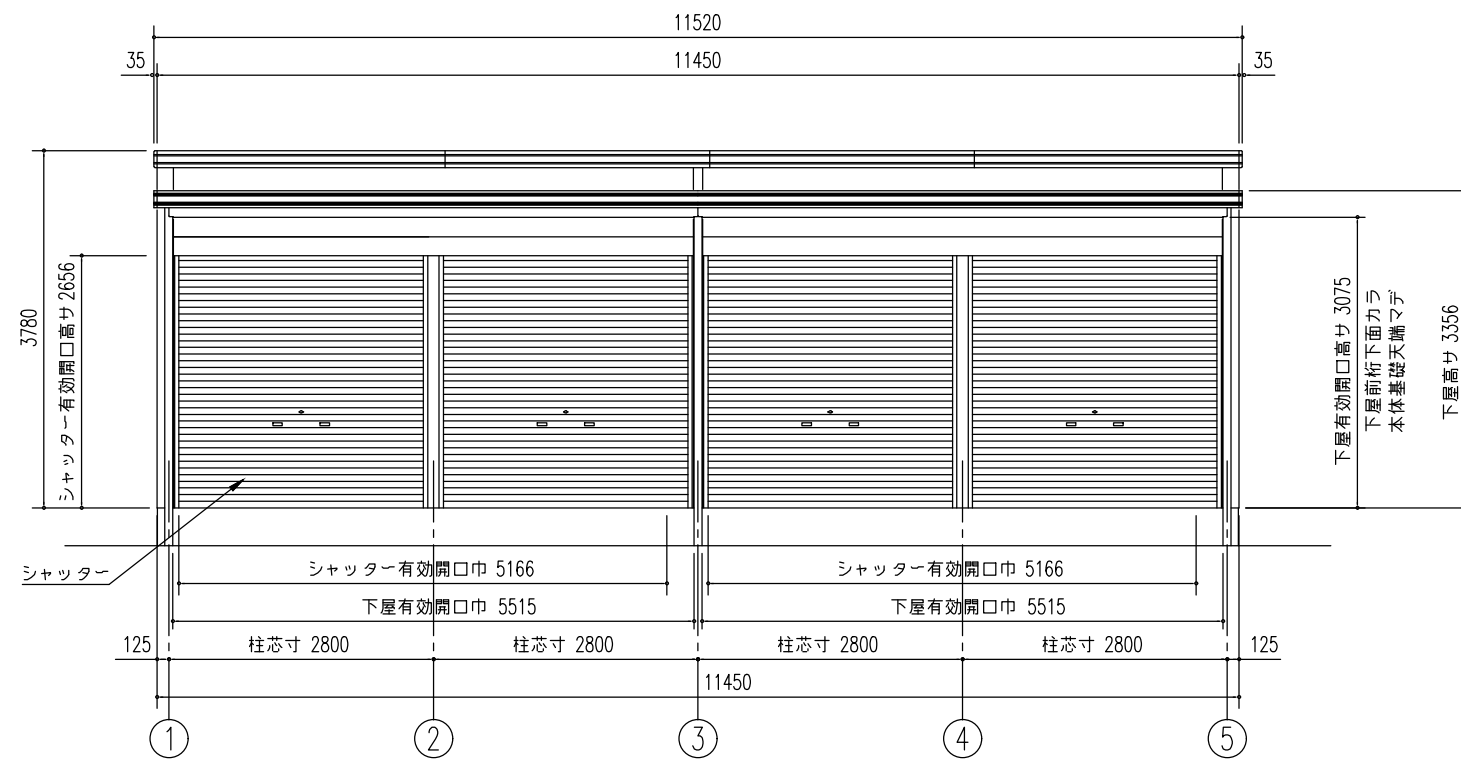
正面立面図(S= 1/80)
