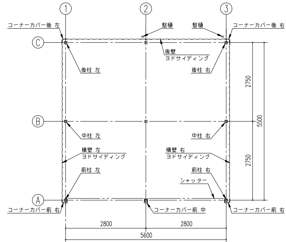
平面図 (S=1/80)
