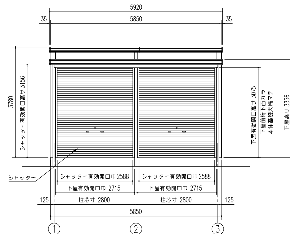
正面立面図 (S=1/80)
