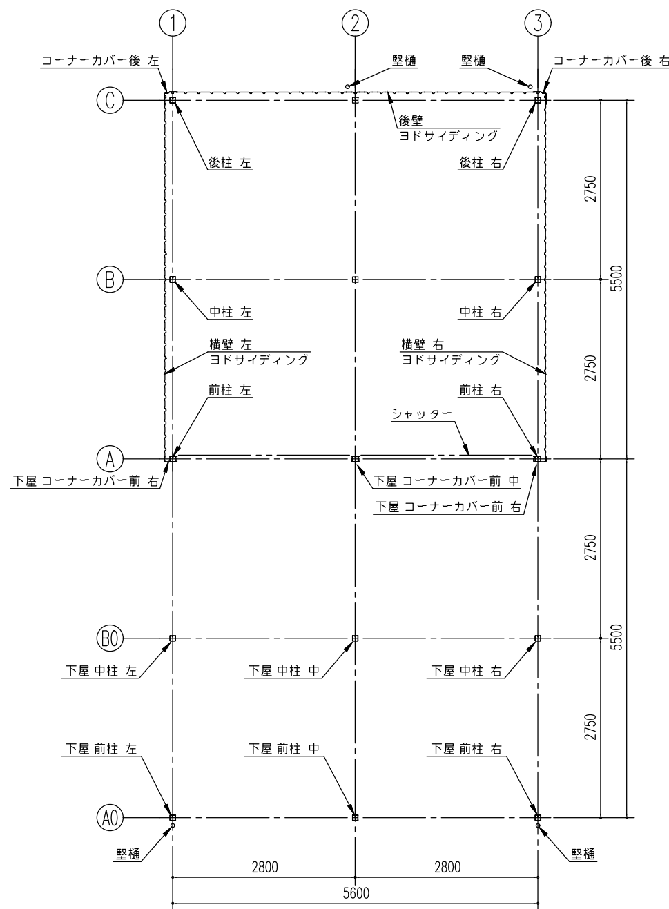
平面図 (S=1/80)
