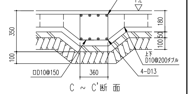
ベタ基礎断面図 (S = 1/20)
