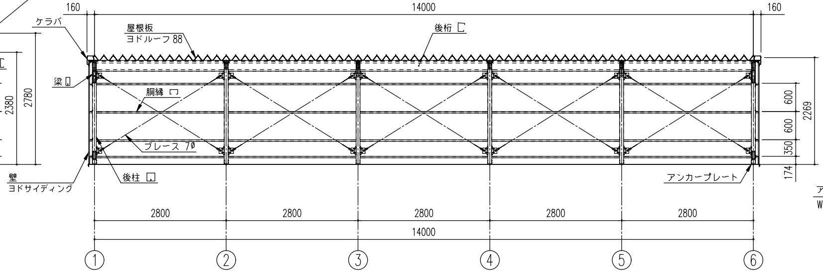
正面断面図 (S=1/80)
