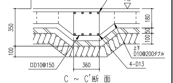
ベタ基礎断面図 (S=1/20)
