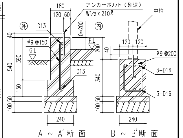
布基礎断面図 ( S = 1/20 )
