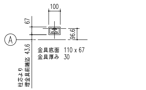
埋金具詳細図 (S = 1/20)
