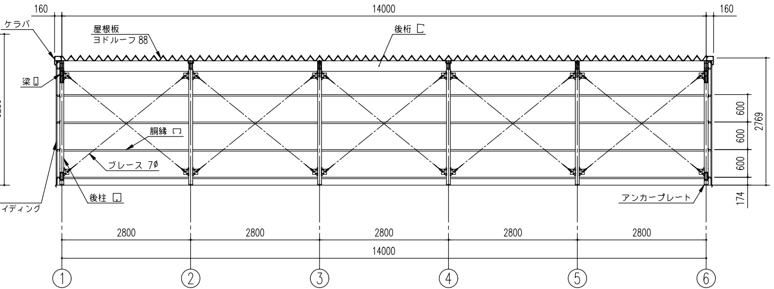
正面断面図 (S= 1/80)
