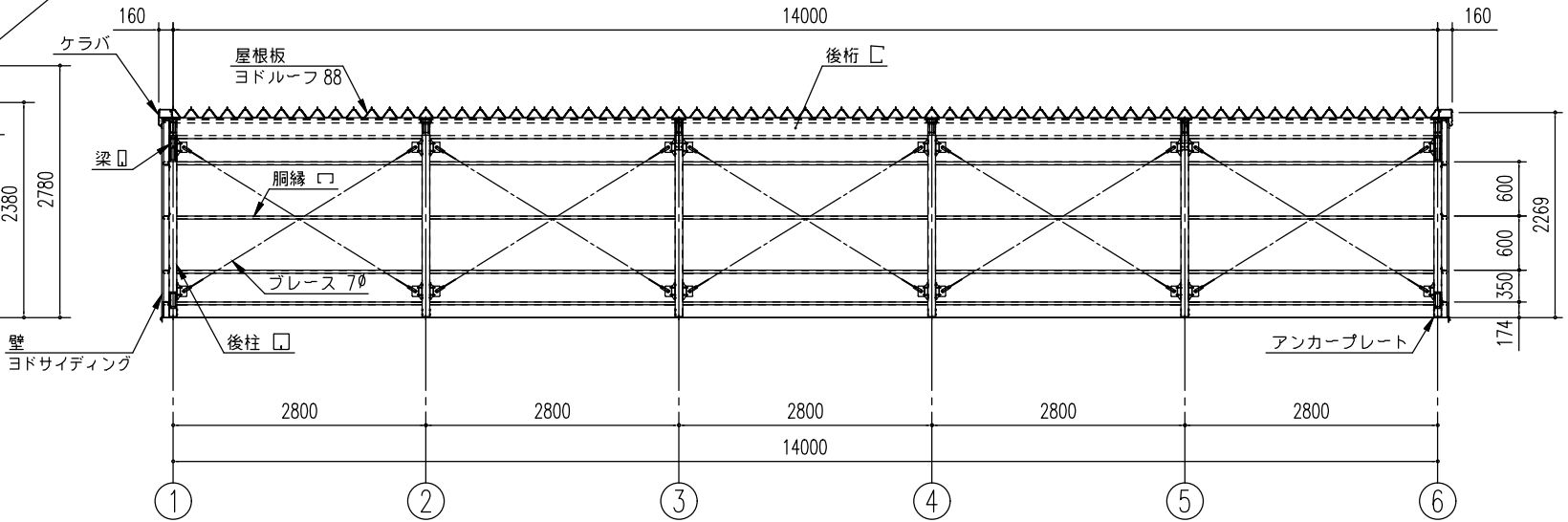
正面断面図 (S= 1/80)
