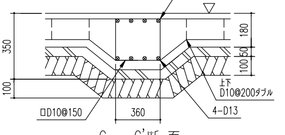
C ~ C' 断面
