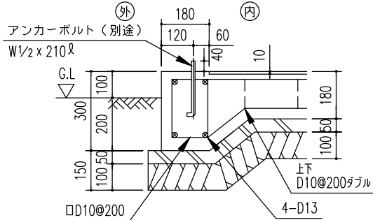
A ~ A' 断面
