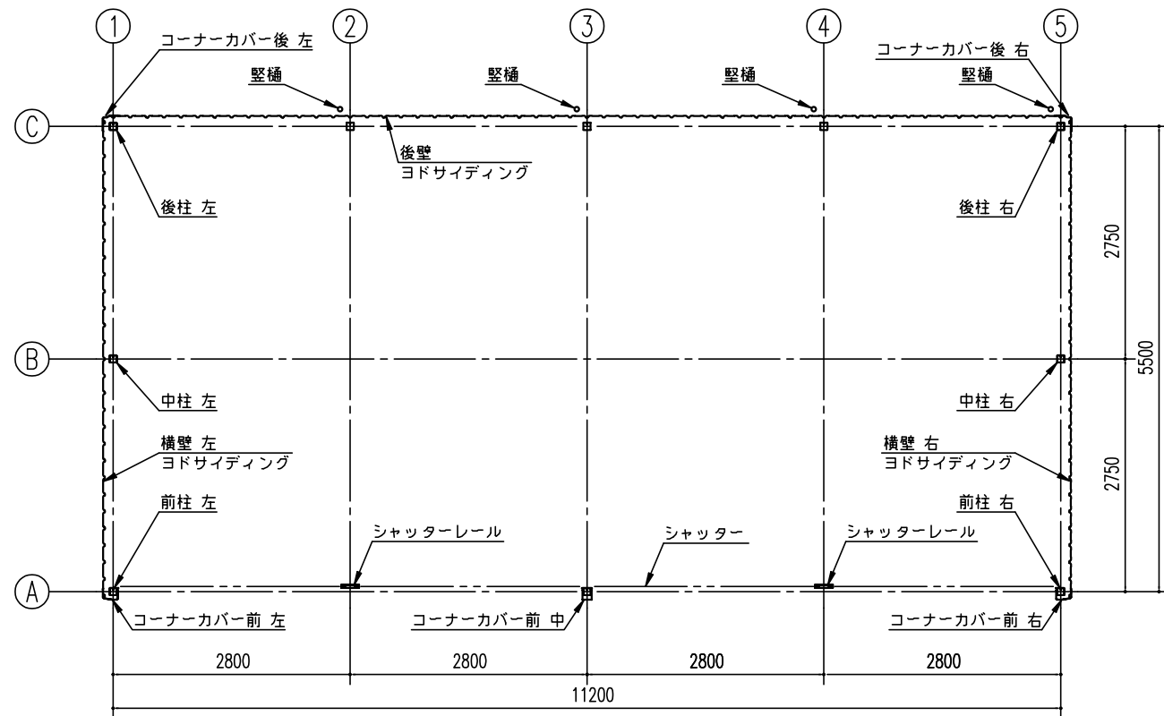
平面図 (S=1/80)
