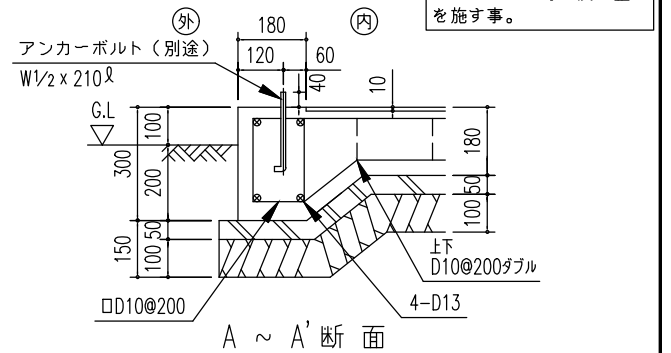
埋金具詳細図 (S = 1/20)
