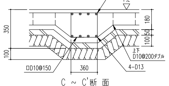
ベタ基礎断面図 (S = 1/20)
