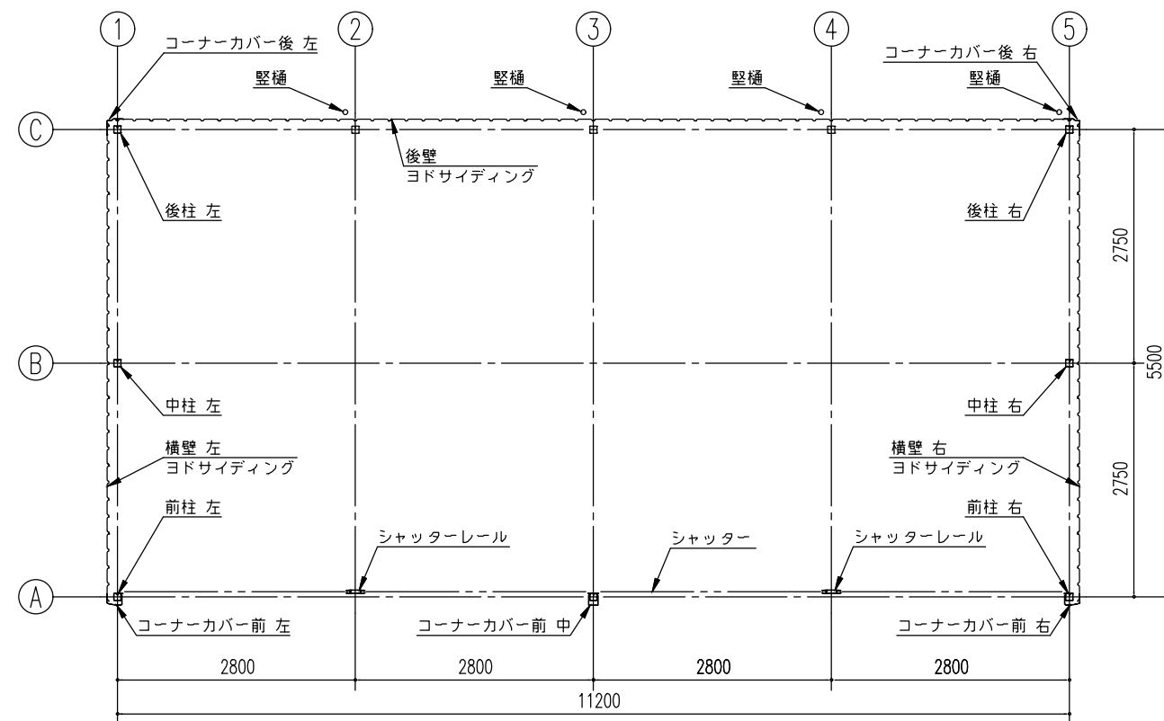
平面図 (S=1/80)
