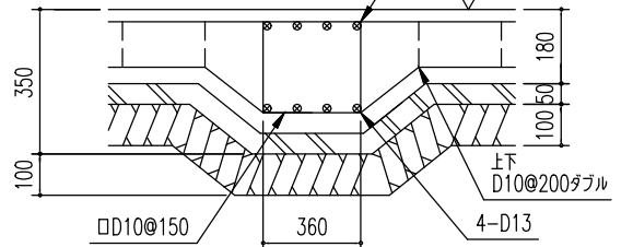
C ~ C'断面
