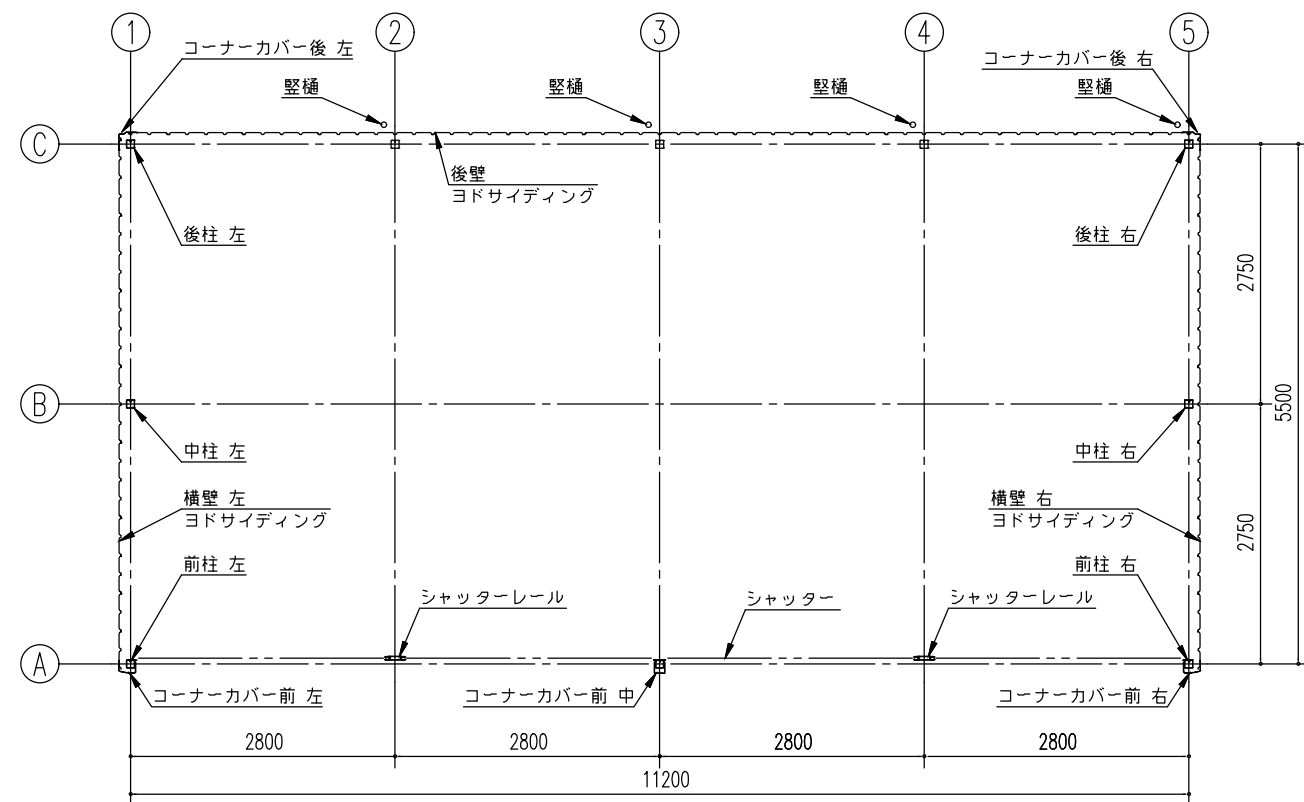
平面図 (S=1/80)
