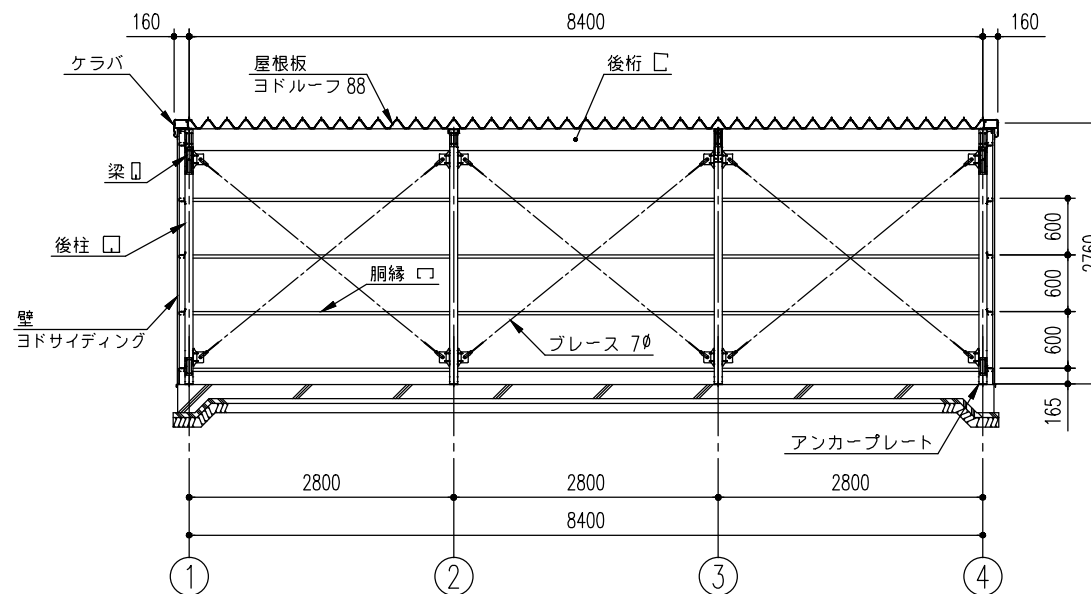
本体 正面断面図 (S=1/80)
