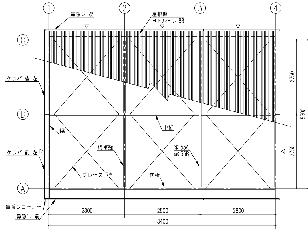
小屋伏図 (S=1/80) ▷は、プレース 7φ とする。
