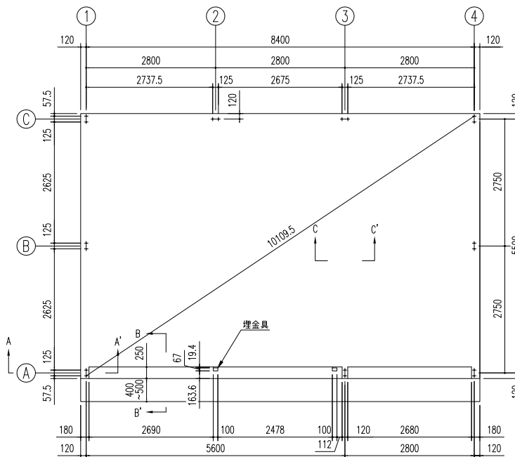
基礎伏図 (S=1/80)
