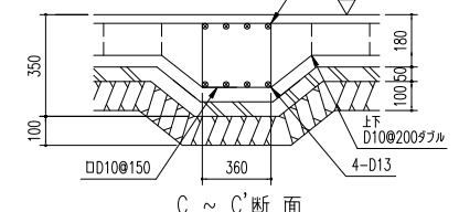
C ~ C' 断面
