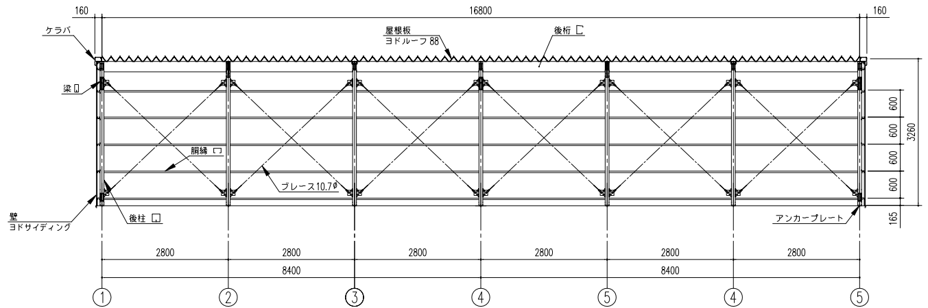
正面断面図 (S=1/80)
