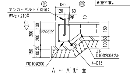
埋金具詳細図 (S=1/20)
