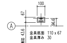
埋金具詳細図 (S=1/20)
