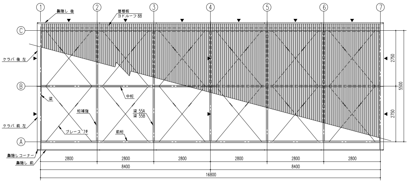
小屋伏図 ▶は、プレース 10.7φ とする。
