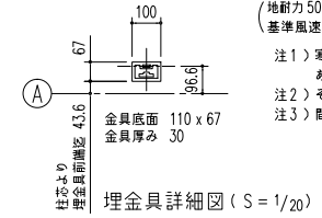
埋金具詳細図 (S=1/20)
