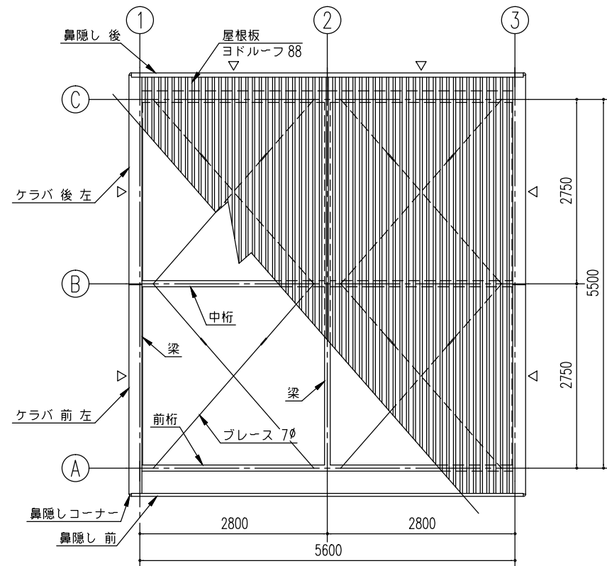
小屋伏図 (S=1/80) ▷は、ブレース 7° とする。
