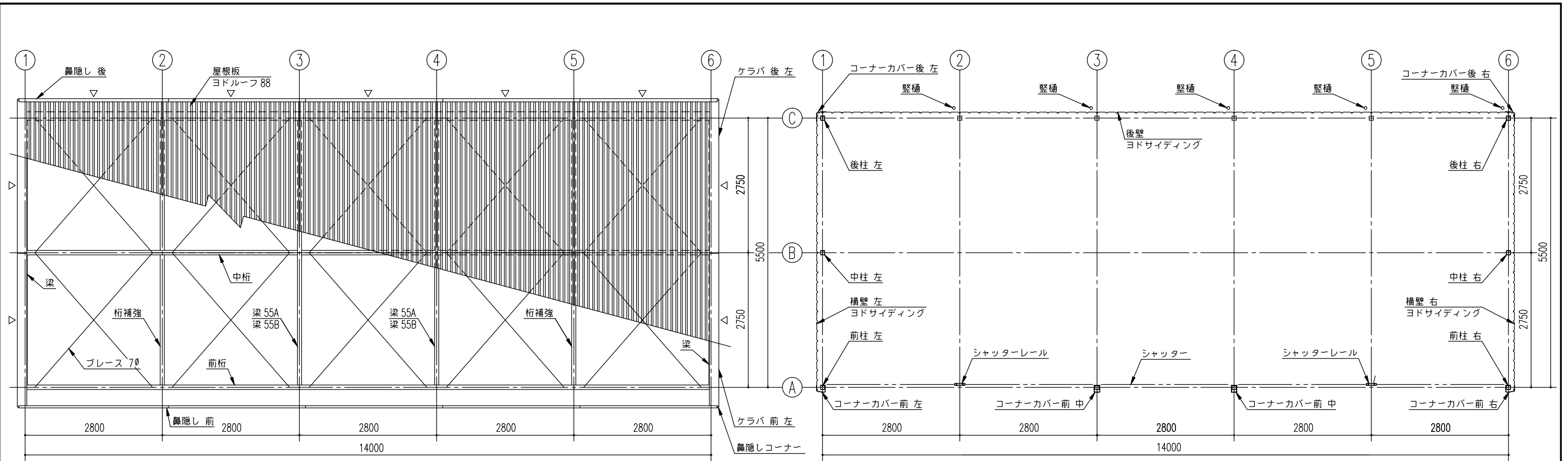
△は、ブレース7φとする。
