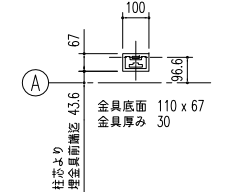
埋金具詳細図 (S=1/20)
