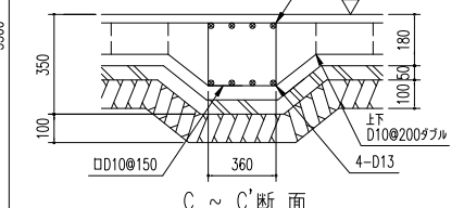
C ~ C' 断面
