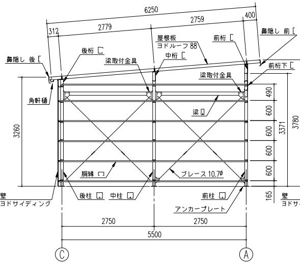
側面断面図 (S=1/80)
