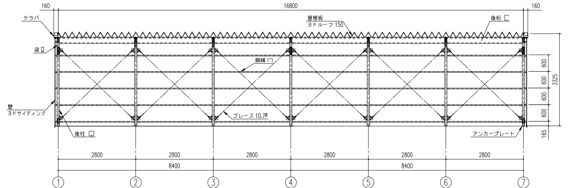
正面断面図 (S=1/80)
