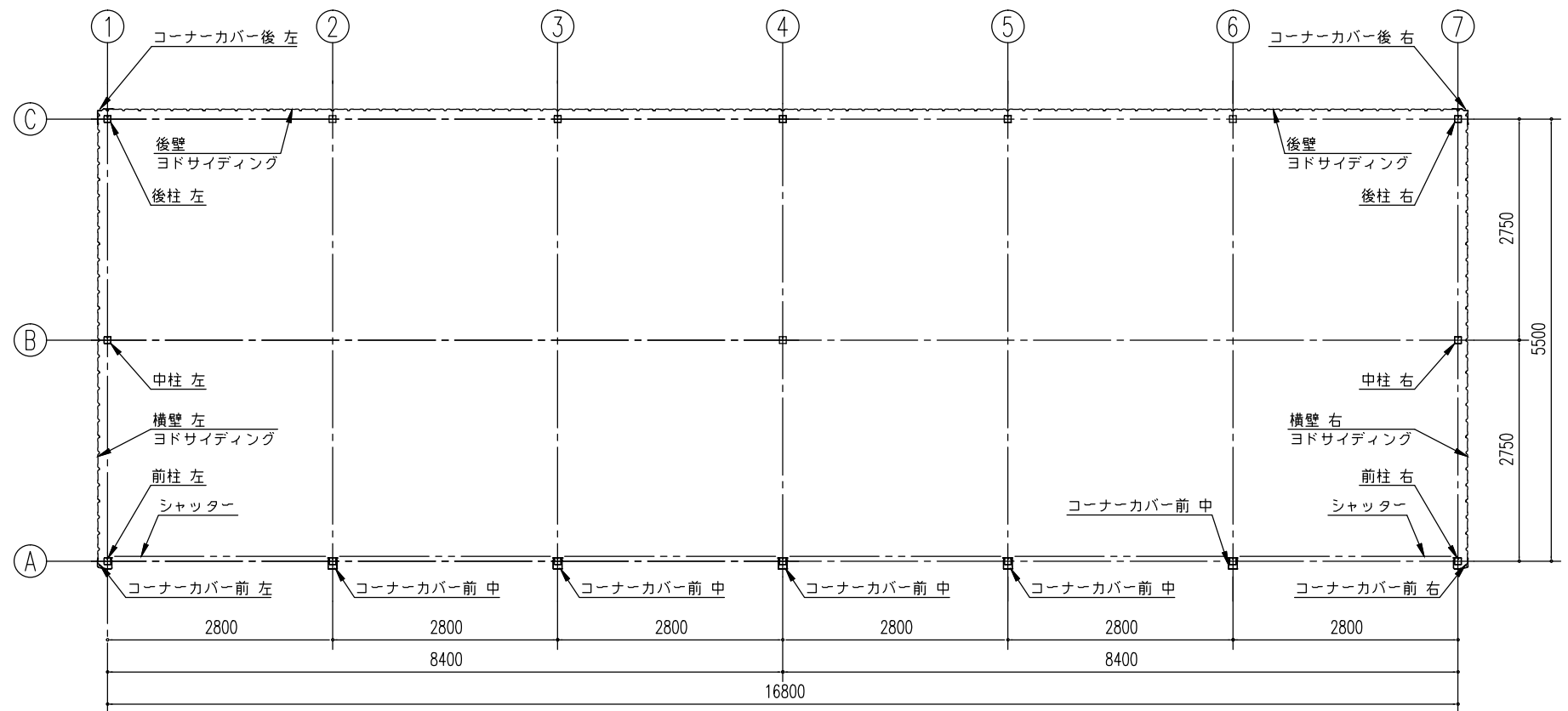
平面図 (S=1/80)
