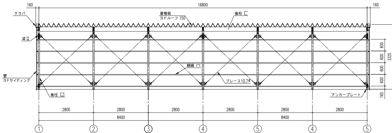
正面断面図 (S=1/80)
